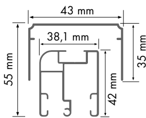
COULISSE SUPÉRIEURE
